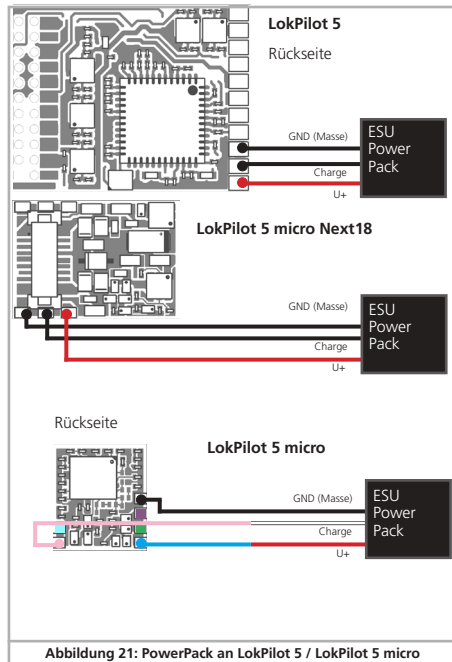
Abbildung 21: PowerPack an LokPilot 5 / LokPilot 5 micro
