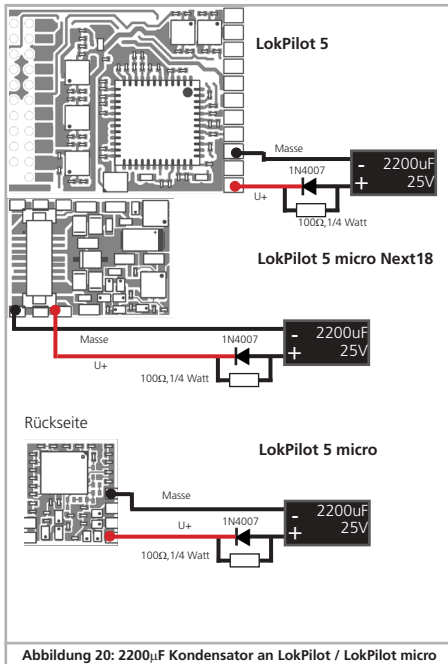
Abbildung 20: 2200µF Kondensator an LokPilot / LokPilot micro
