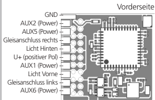
Abbildung 8: LokPilot 5 Fx & LokPilot 5 Fx DCC mit 8-poliger NEM652 Schnittstelle
