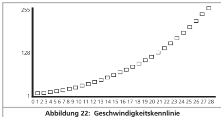
Abbildung 22: Geschwindigkeitskennlinie
